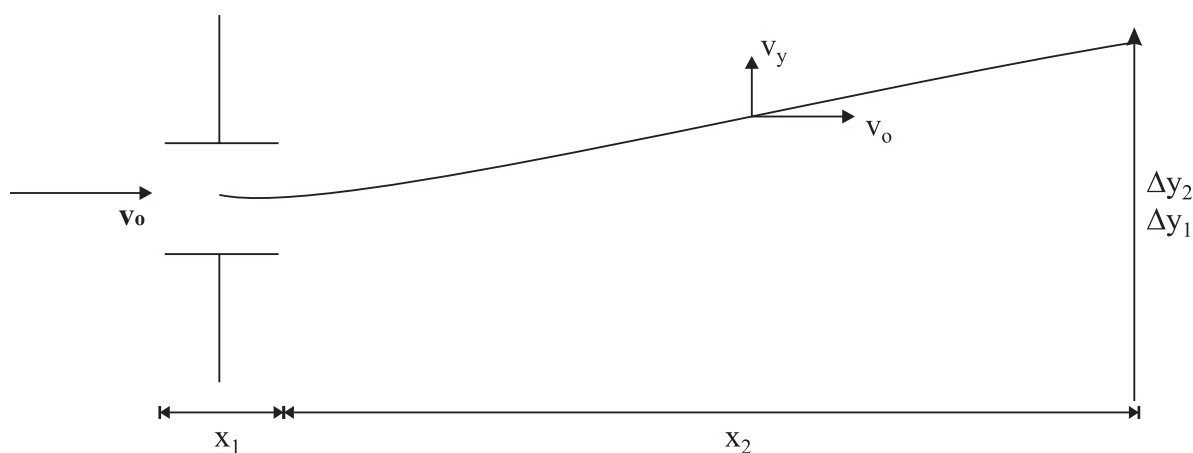
Figura 6.14: Desvio das partículas carregadas
