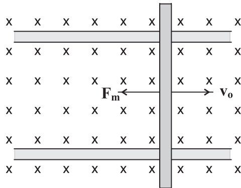
Figura 6.52: Barra deslizando em campo magnético
