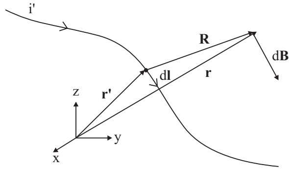
Figura 6.15: Elemento de Campo Magnético
