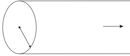
Figura 6.38: Direção da densidade de corrente
