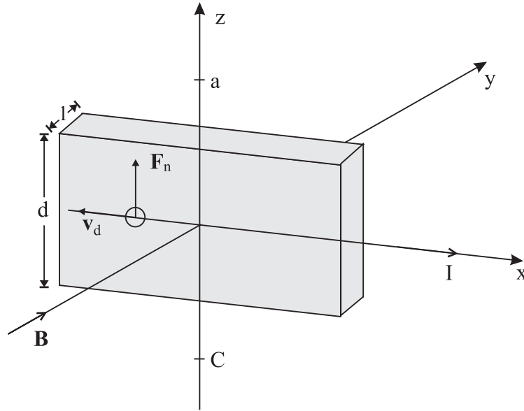
Figura 6.12: Efeito Hall
